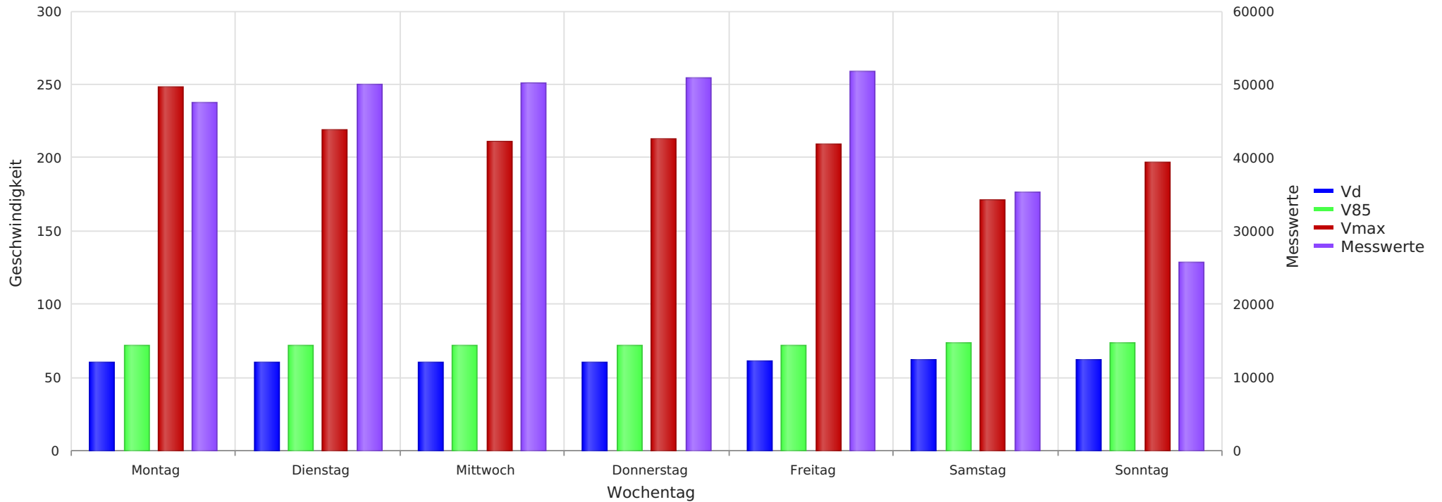
Rudelzhausen Schoosfeld, ortseinwärts, 50 km/h Beschränkung Vd, V85, Vmax, Anzahl der Messwerte vs. Wochentag
